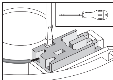
Způsob zapojení vodičů.
