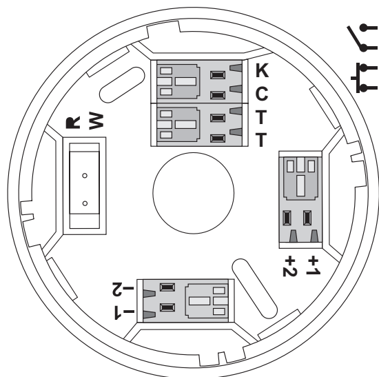
Svorky detektoru
