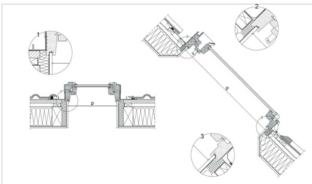
Princip měření vnitřních světých rozměrů ostění (rozteče SDK drážek) u starého okna.
